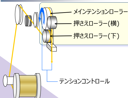
ワイヤ放電加工機の送給系模式図
